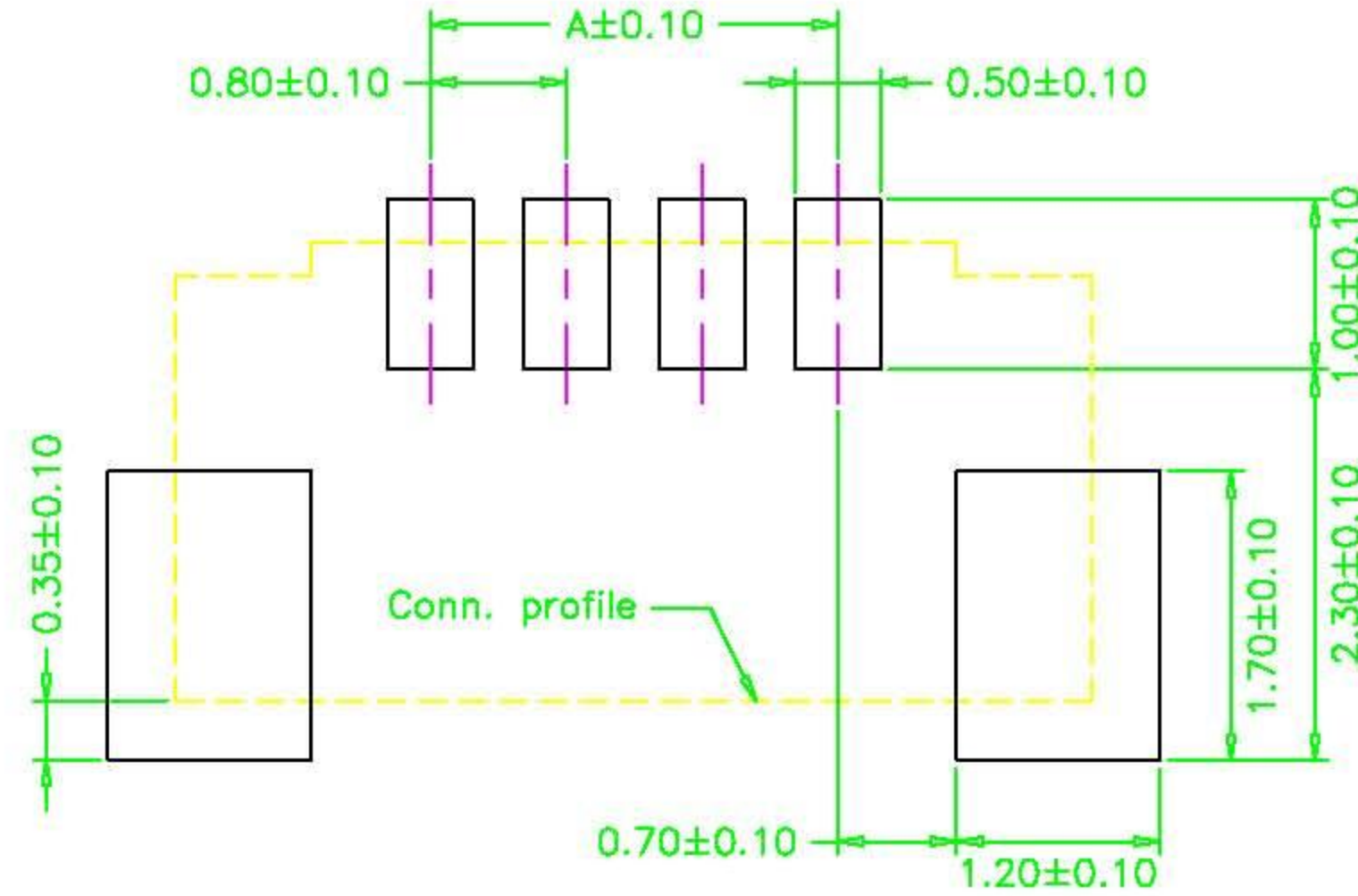
P.C.B. LAYOUT
